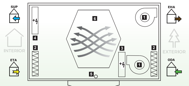
Linker versie - bovenaanzicht
