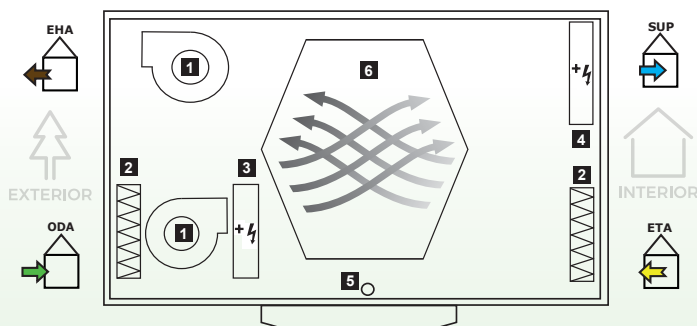
Rechter versie - bovenaanzicht
